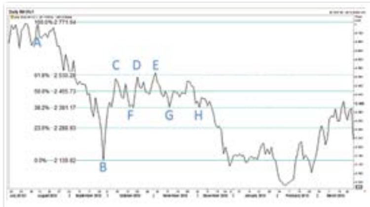
Grafiek 1. Fibonacci-Terugtrekking
