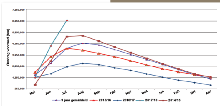
Grafiek 3. Die oordragvoorraad van witmielies per maand in Suid-Afrika oor bemarkingsjare (Sagis).
