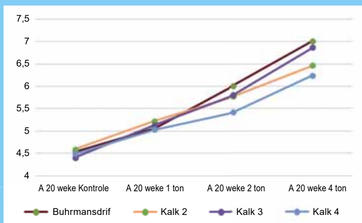
Grafiek 2: Die pH-verhoging op 20 weke gemeet van Buhrmansdrif-kalsiet teen ander kalsietbronne.
